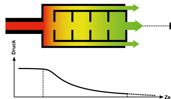
RBS Schalldämpfer
